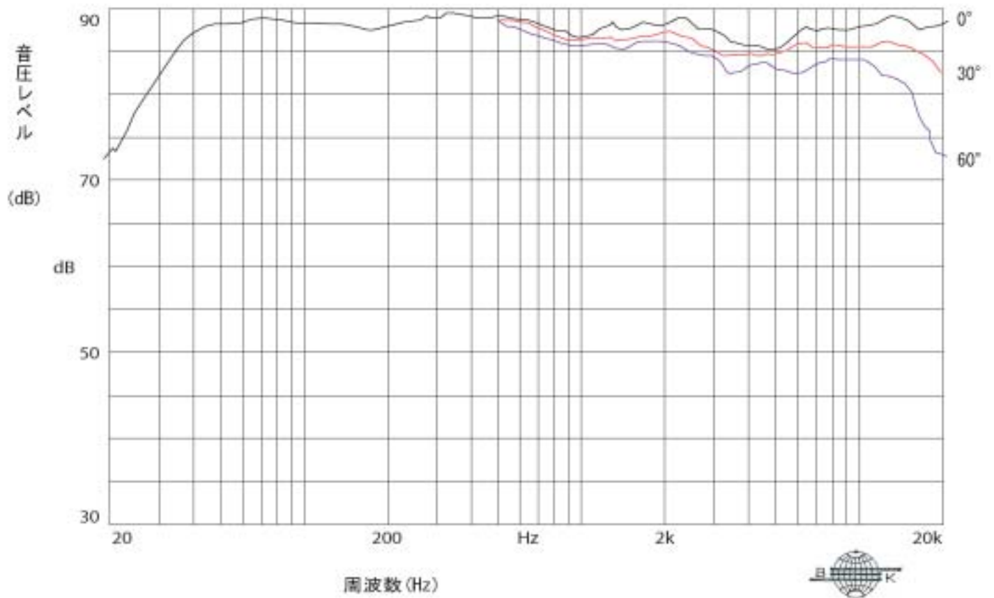
KX-1000P指向特性 ( 0° , 30° , 60° )
