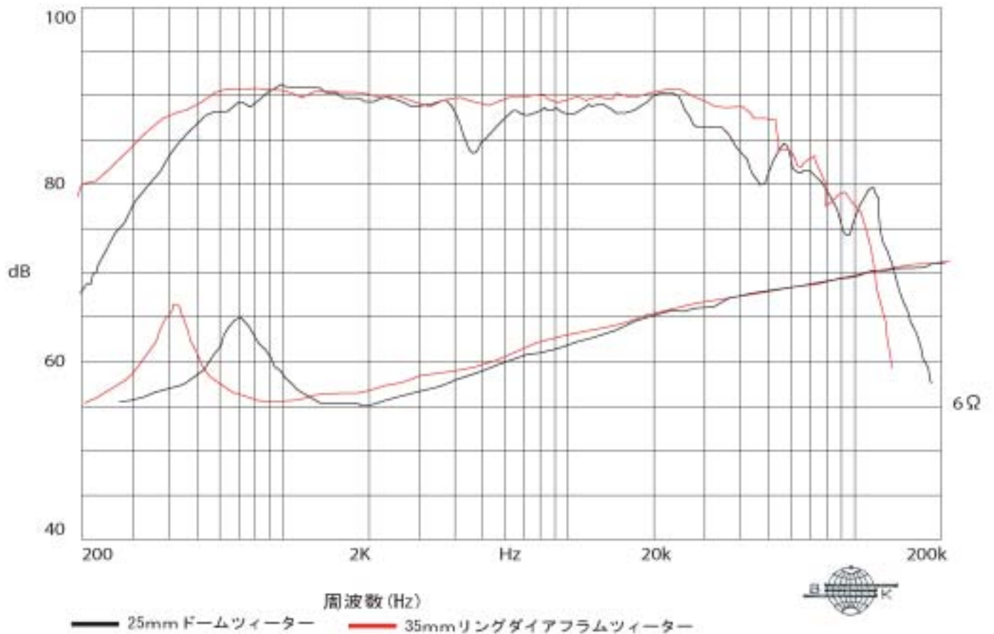
KX-1000P 25mmドームツイーターと35mmリングツイーターの比較
