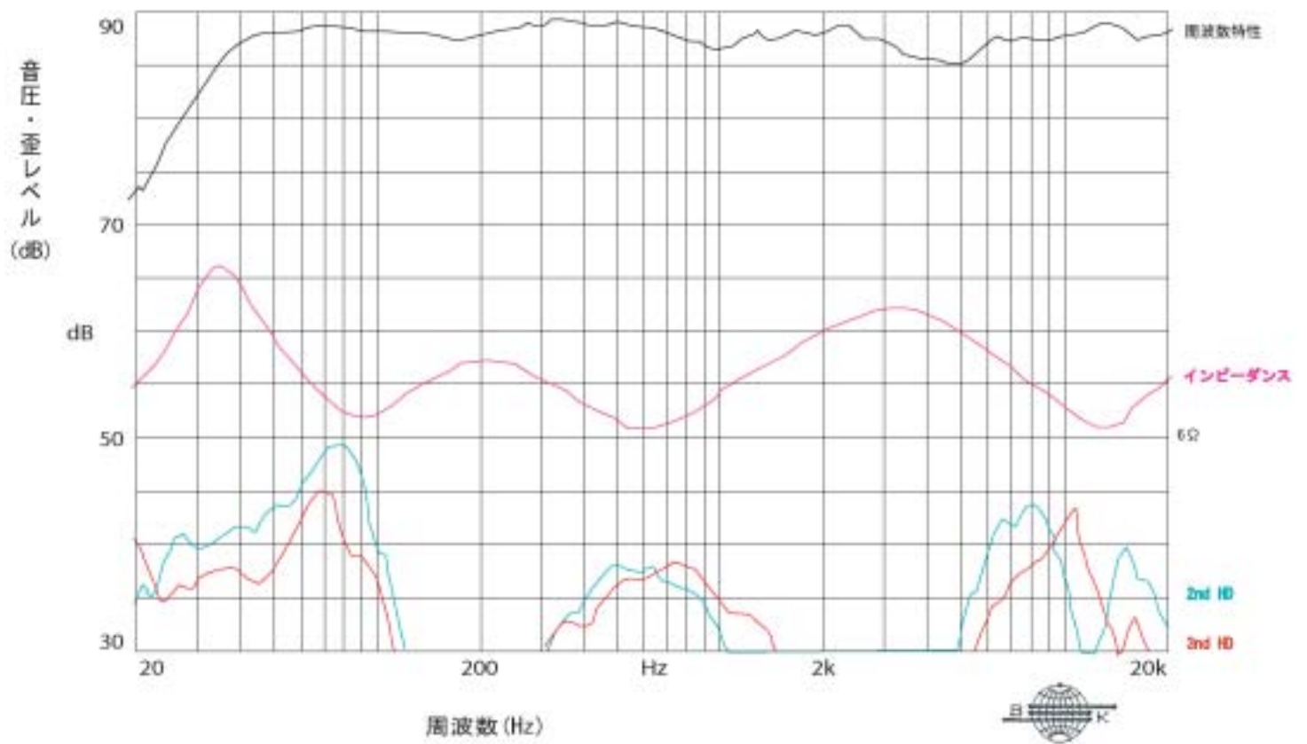
KX-1000P音圧・歪・インピーダンス特性
